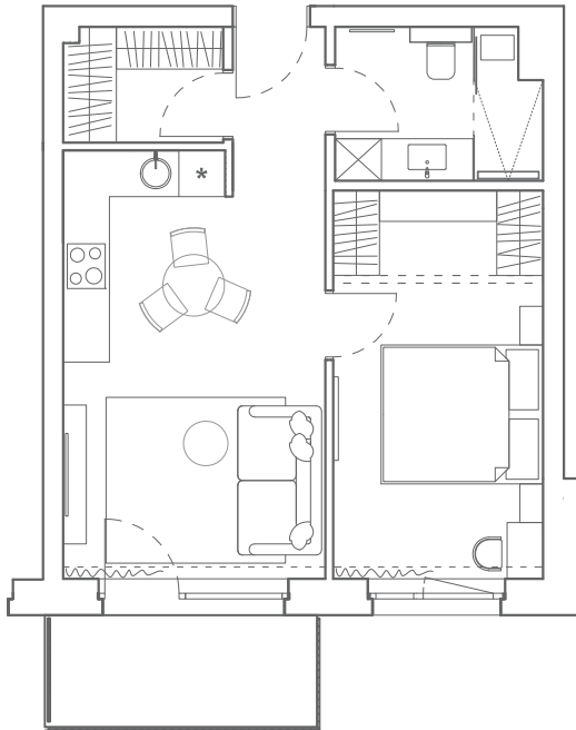
BUTO BALDŲ IŠDĖSTYMO PLANAS
